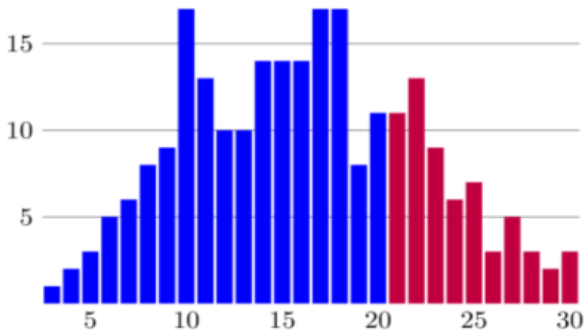
Рис. 3: Проект ABC@home находит все тройки ABC чисел для заданной верхней границы «качества» q_{ABC} и числа десятичных разрядов.
